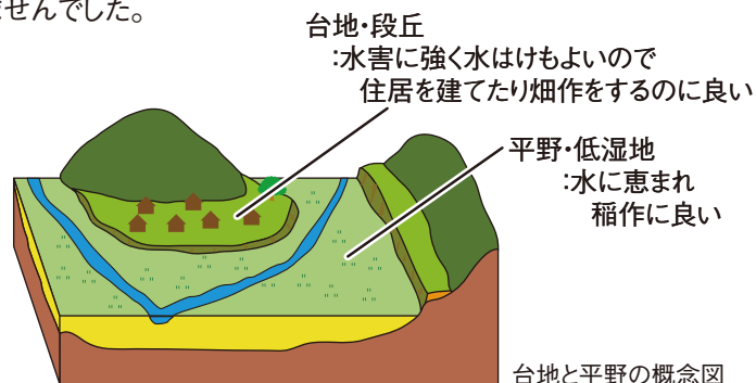
台地と平野の概念図
