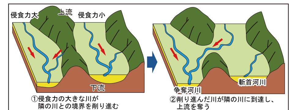
河川争奪概念図
